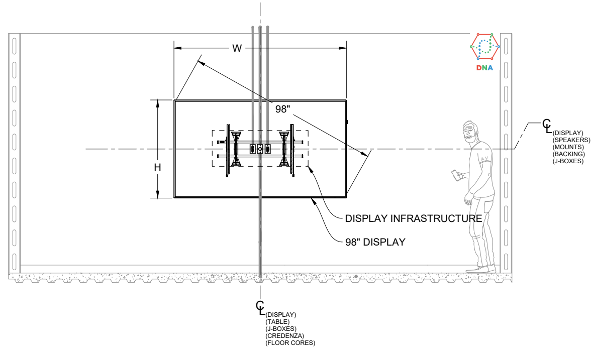
1 98" DISPLAY - ELEVATION DNADT-02 SCALE: 1/4" = 1'-0"
